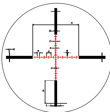
G28 MIL DOT RETICLE SUBTENSION
